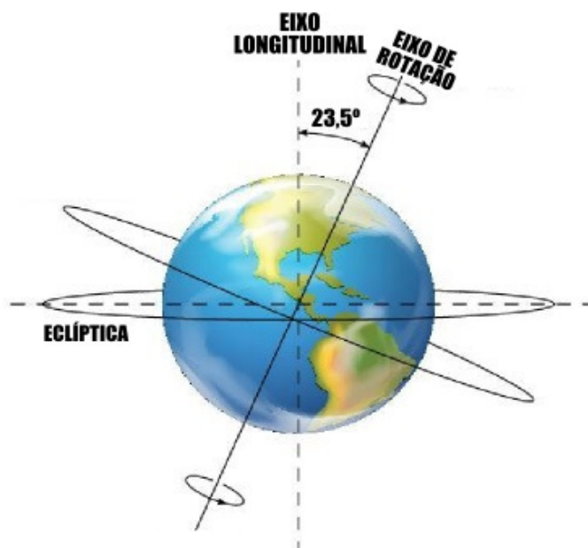
Figura 3.4 - Inclinação da Terra.
